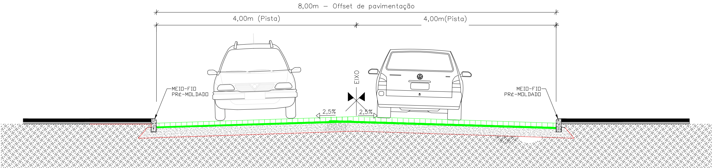
SEÇÃO TIPO DE PAVIMENTAÇÃO- Offset de pavimentação com bloco intertravado-Rua Trav. Professor Antônio Balthazar Englert
